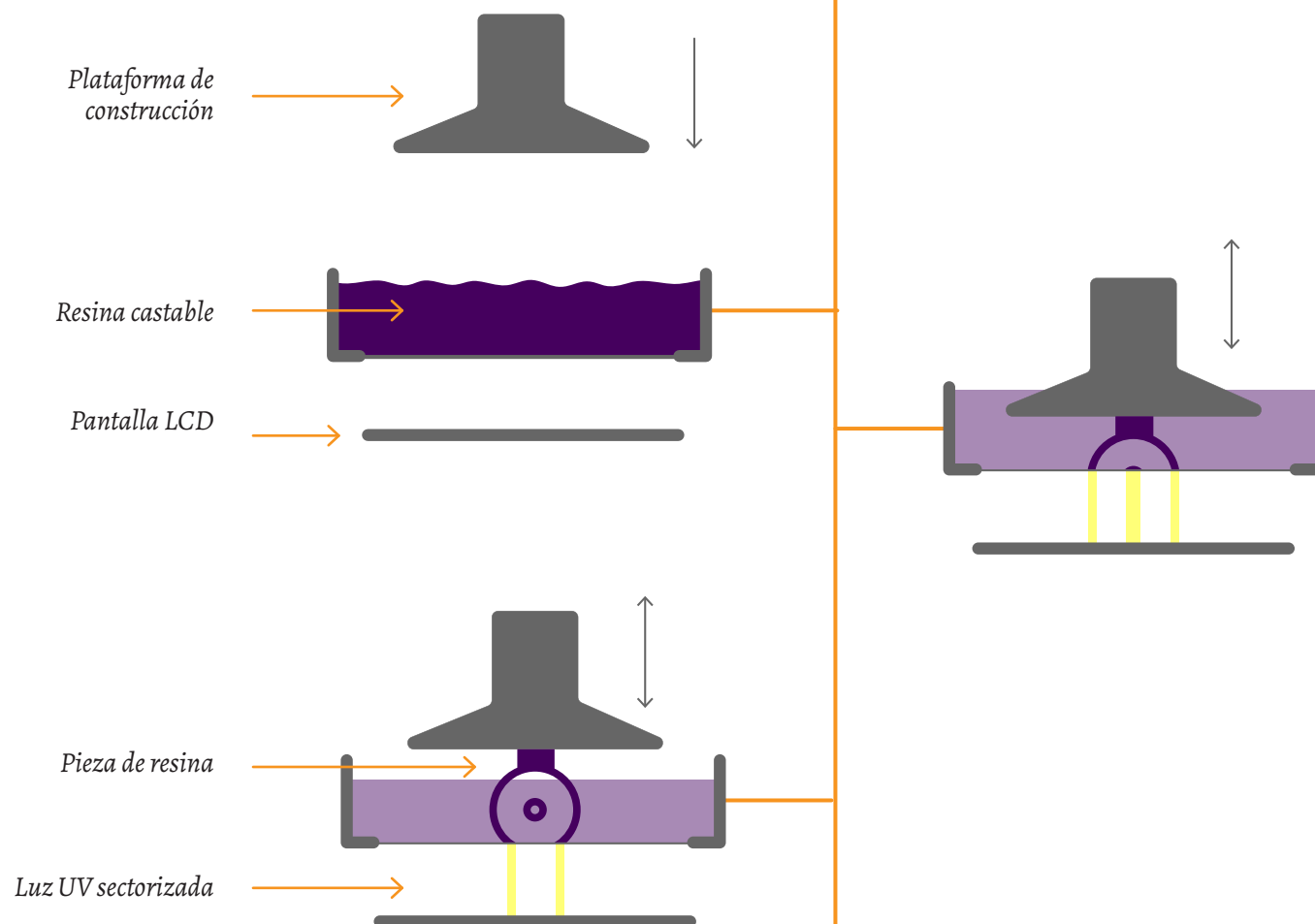
Figura 9. Etapas de impresión 3D, basada en Zoffli Momberg, 2021. Elaboración propia, 2023.
