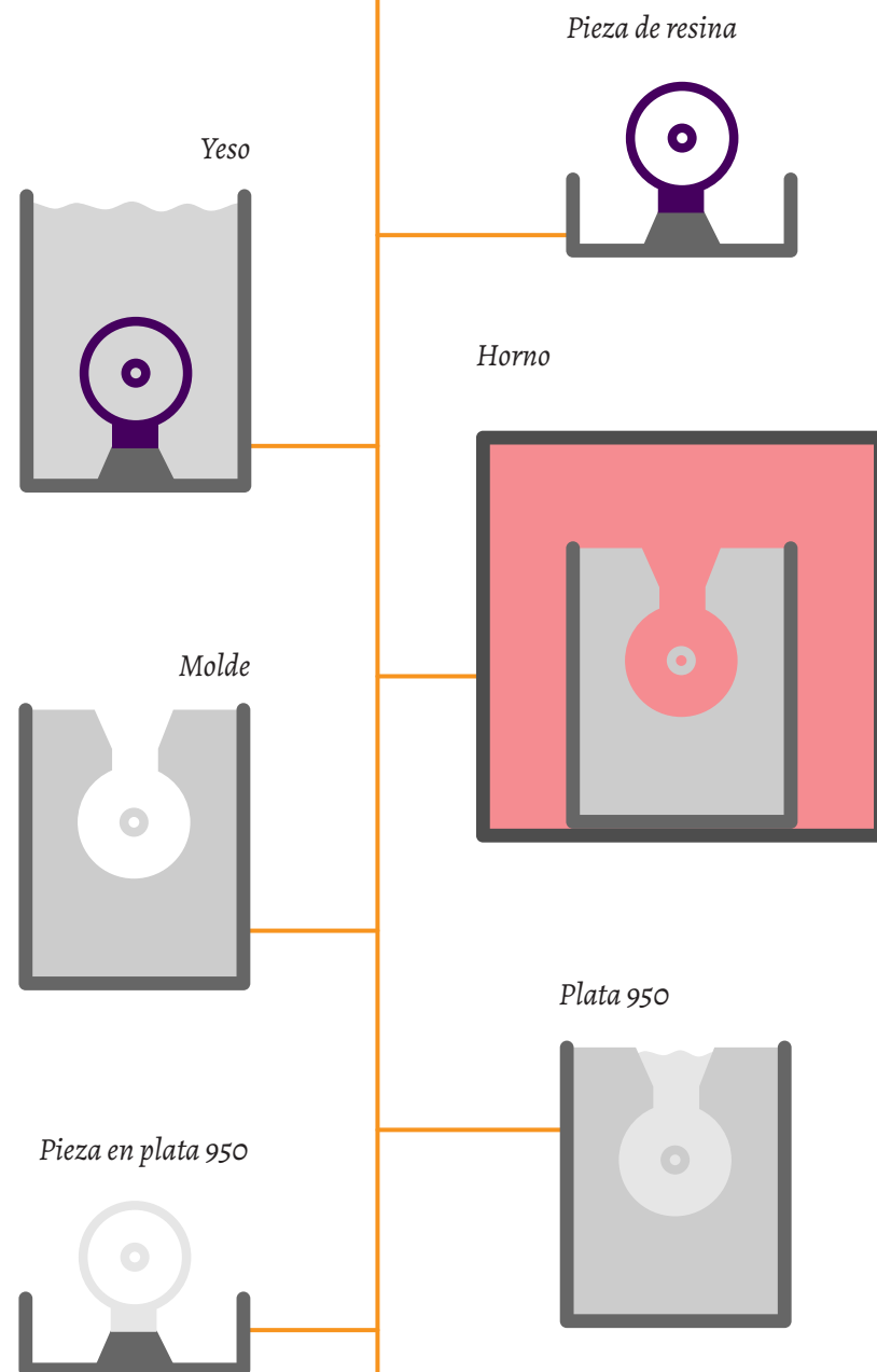
Figura 10. Etapas casting de joyas, basada en Zoffli Momberg, 2021. Elaboración propia, 2023.
